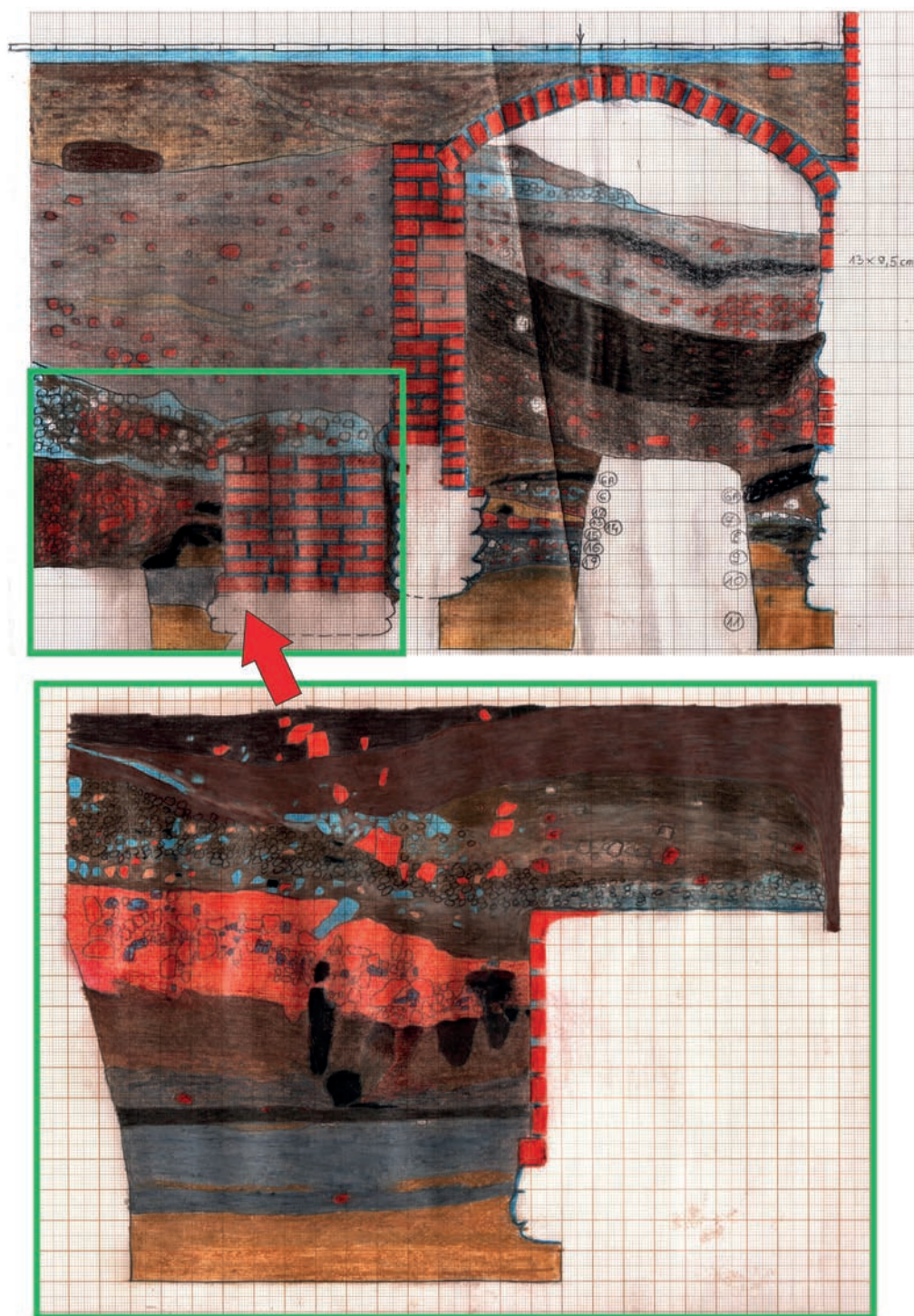
Ryc. 14. Opactwo cystersów w Mogile. Przekrój ceglano punktowego z połowy XIII w. z relikami spalonej konstrukcji szachulcowej i glinianym klepiskiem podłogi odkrytymi podczas badań archeologicznych w zachodniej części przeoratu (szczegółowy rysunek z elementami konstrukcji z XIII w. u dołu narysowany po pionowym przycięciu profilu). Rys. D. Niemiec i J. Olbrot
